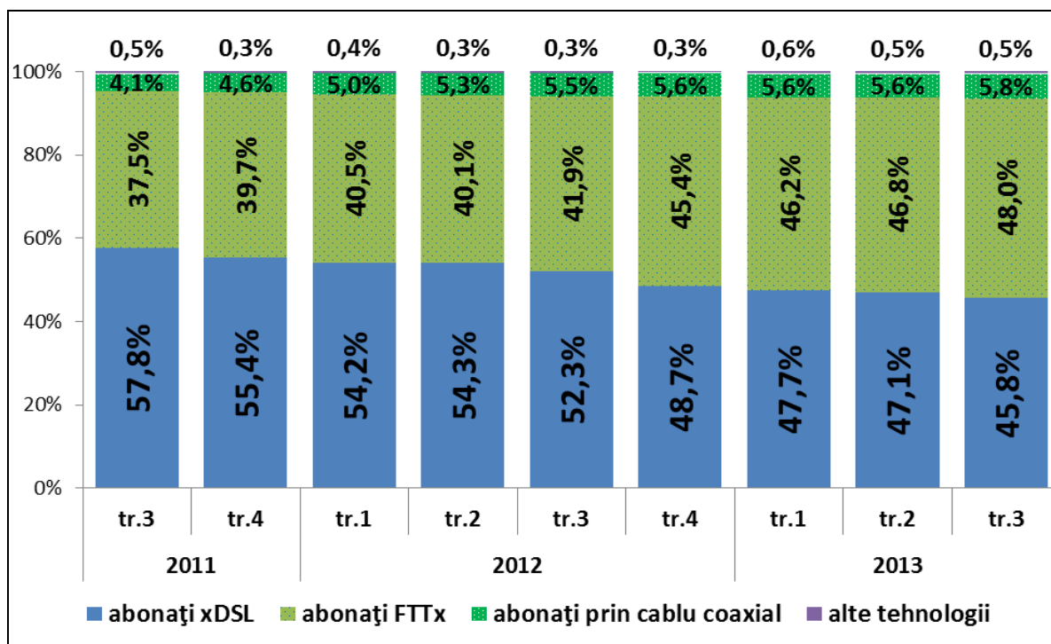
Figura 36. Structura pieței serviciilor în bandă largă în funcție de tehnologia de acces
